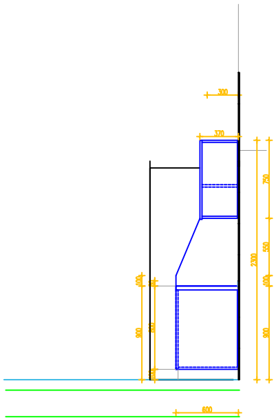
PRESEK E-E
