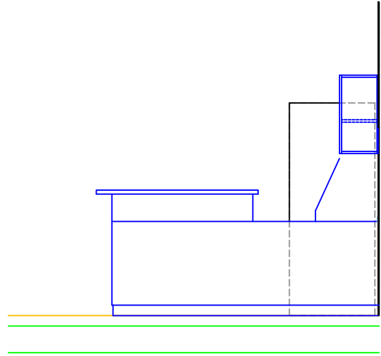
PRESEK D-D
